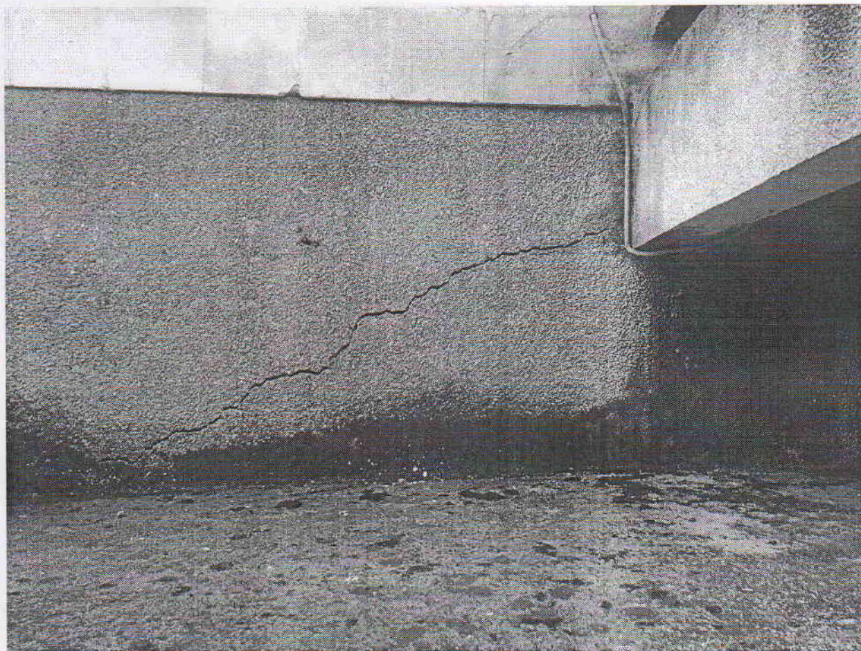
Трещина торцевой стены около входной группы по ул. Шортанова. (гл. фасад)
