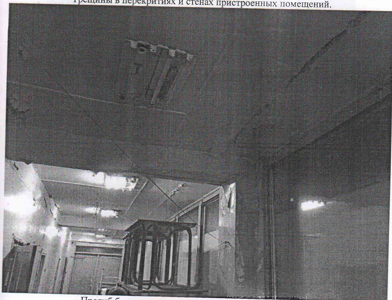
Прогиб балки в коридоре пристроенного помещения.
